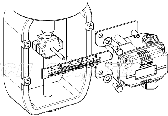
<그림 5> 액추에이터 및 연결봉 조립방법
