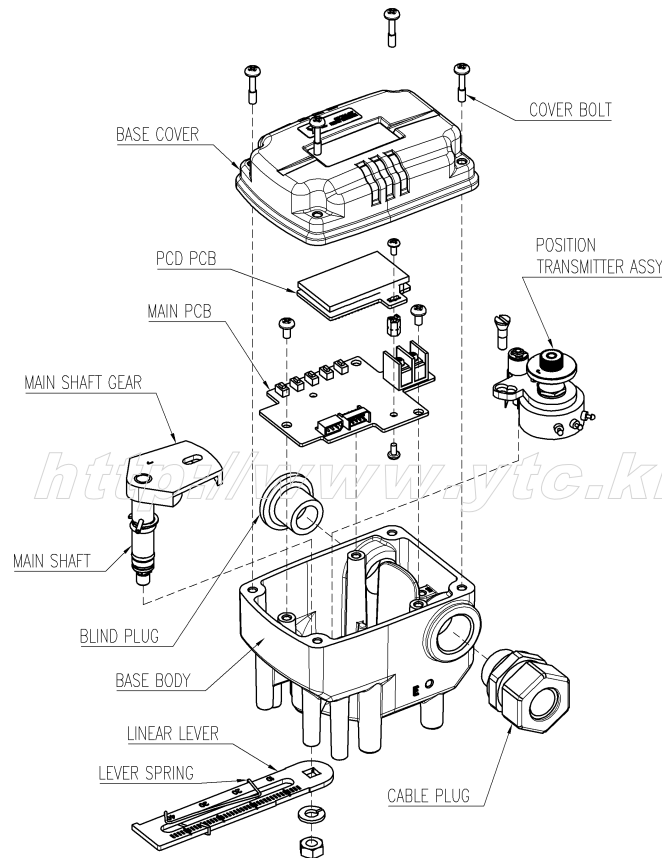
<그림 2> SPTM-5VL내부구조도
