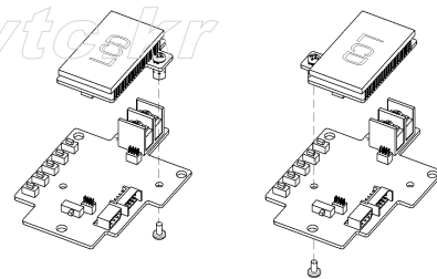
<그림 11> LCD기판의 변경 예
