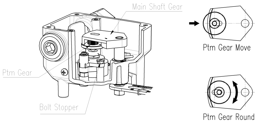
<그림 14> SPTM-5VL의 포텐시오미터 위치 조정
