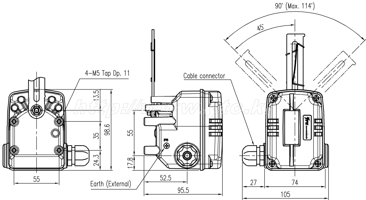
<그림 17> SPTM-5VR 외형도
