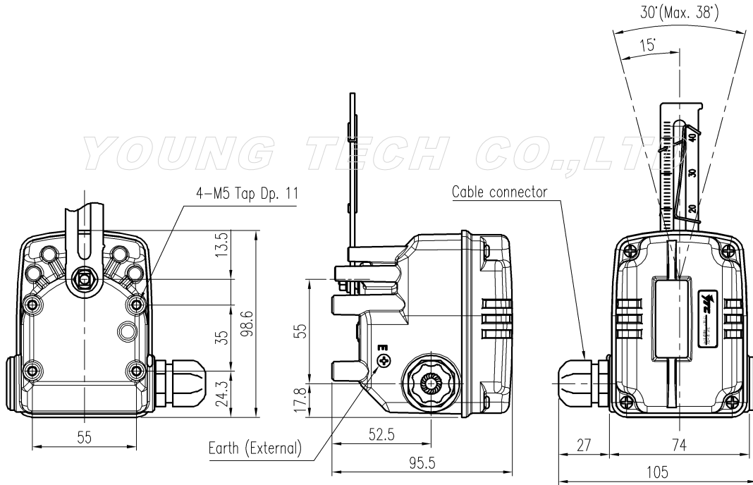
<그림 16> SPTM-5VL 외형도
