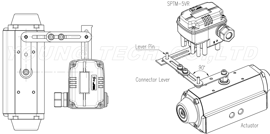
<그림 9> SPTM-5VR의 설치 예
