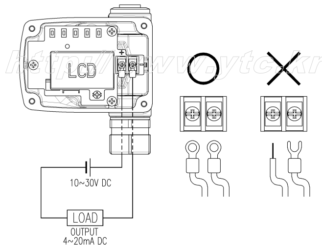
<그림 12> 배선도 및 링형커넥터 연결 예
