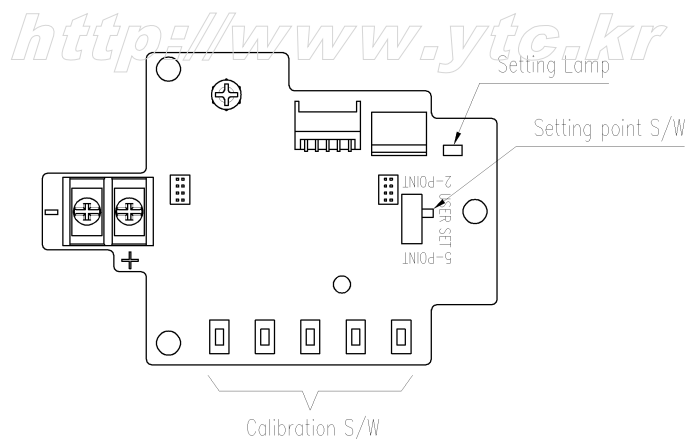
<그림 13> SPTM-5V 기판
