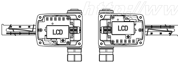
<그림 10> SPTM-5V의 설치방향 예
