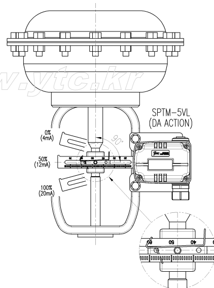
<그림 3> SPTM-5VL 설치
