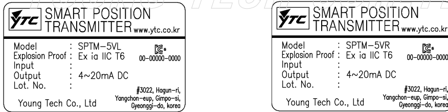
<그림 1> 명판의 표시 (SPTM-5VL, SPTM-5VR)
