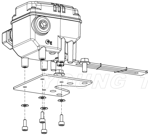
<그림 4> 브라켓 조립방법
