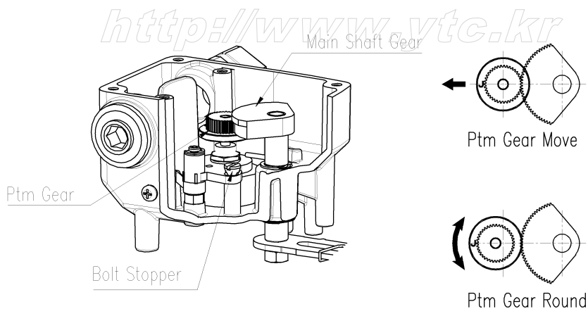
<그림 15> SPTM-5VR의 포텐시오미터 위치 조정
