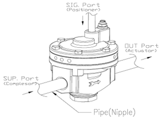
<配管を利用した設置例>
