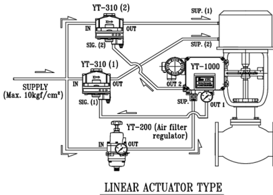
<複動式リニア・シリンダー・アクチュエーターへの設置例>
